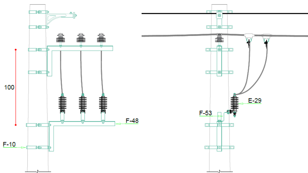
Figura 1 – Estrutura CE2H PR Dimensões em cm
