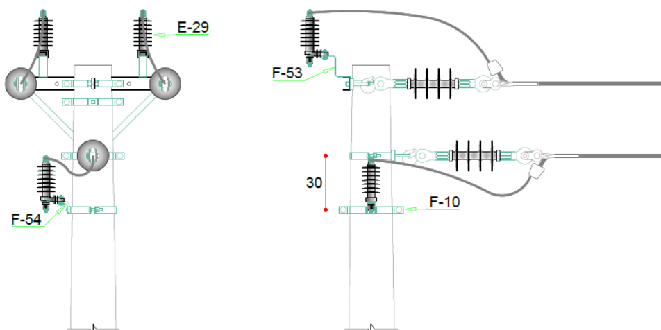
Figura 2 – Estrutura CE3U PR Dimensões em cm
