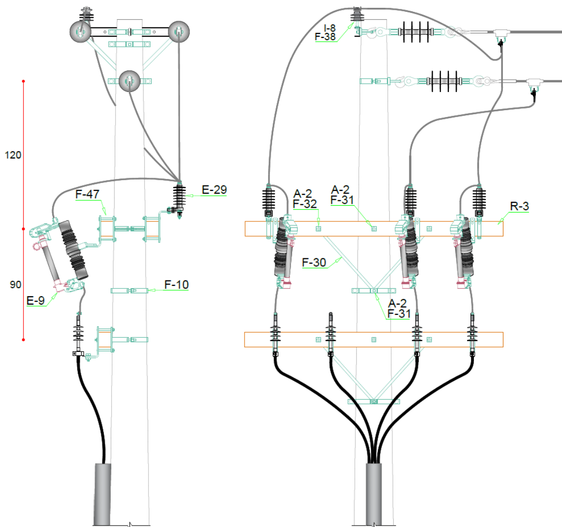
Figura 2 – Estrutura CE3U com entrada subterrânea Dimensões em cm
