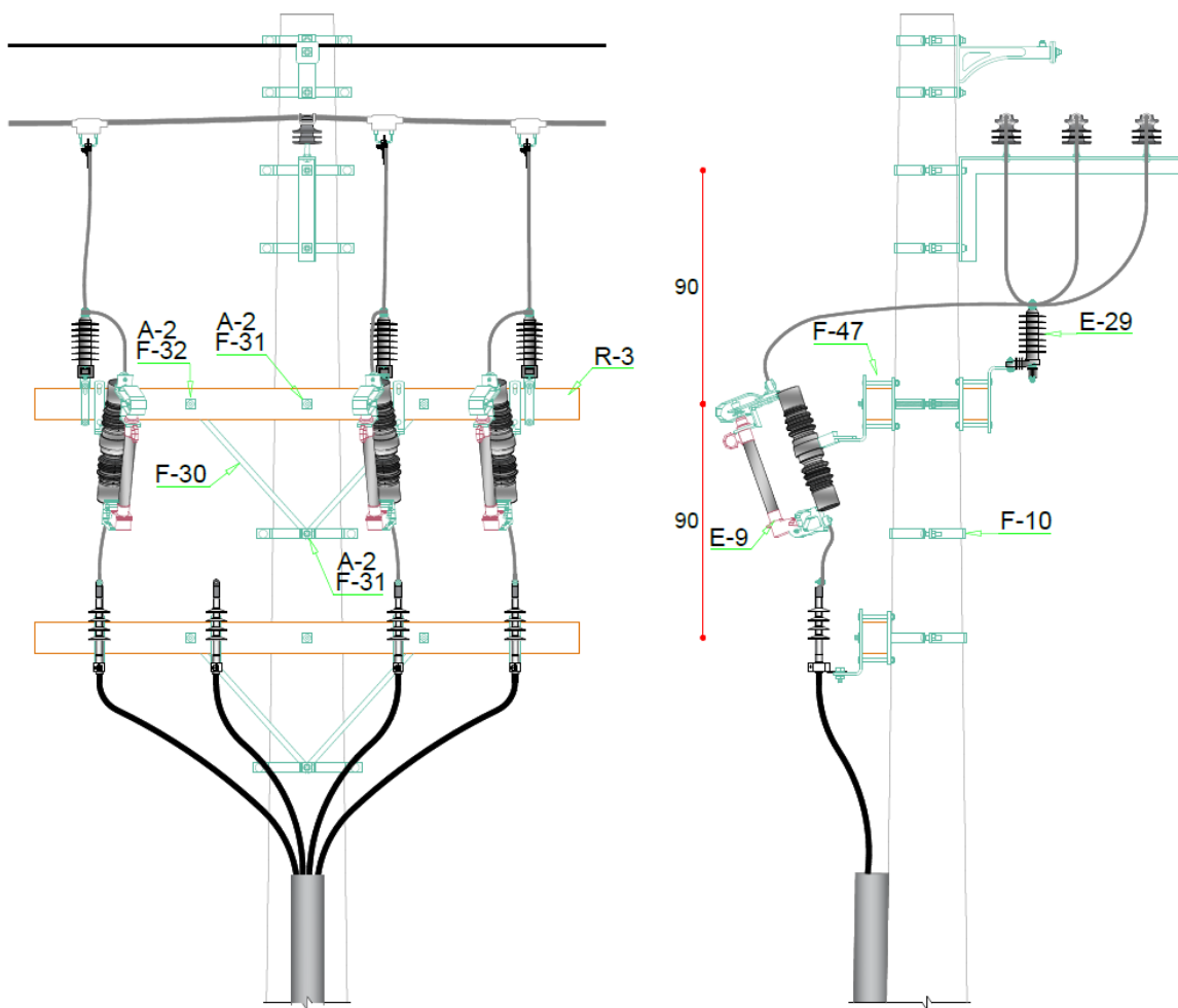
Figura 1 – Estrutura CE2H com entrada subterrânea
