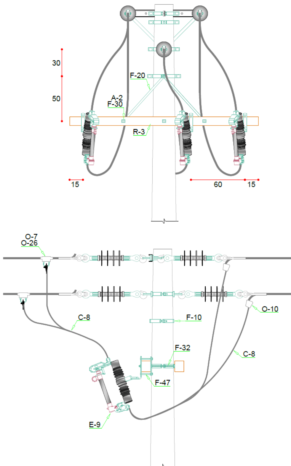
Figura 4 – Estrutura CE4U CF com Perfil U Dimensões em cm
