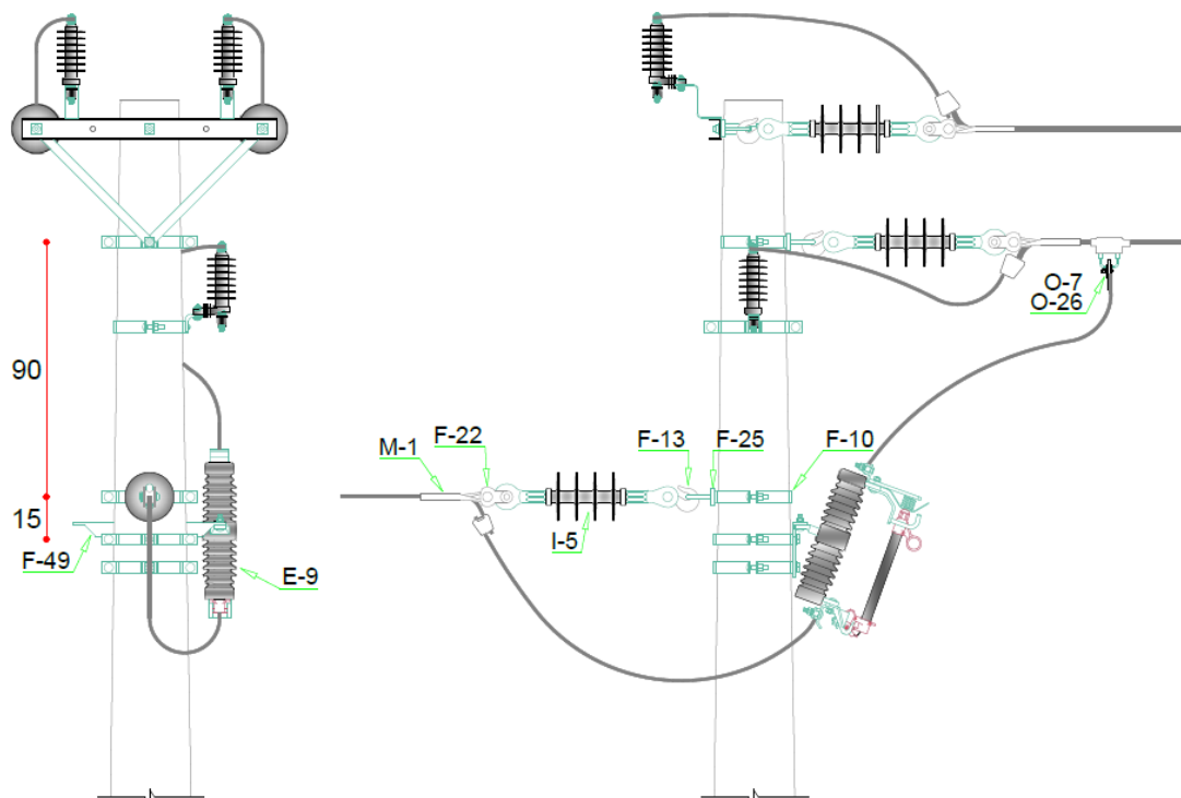
Figura 3 – Estrutura CE3.PR-UP3.CF Dimensões em cm
