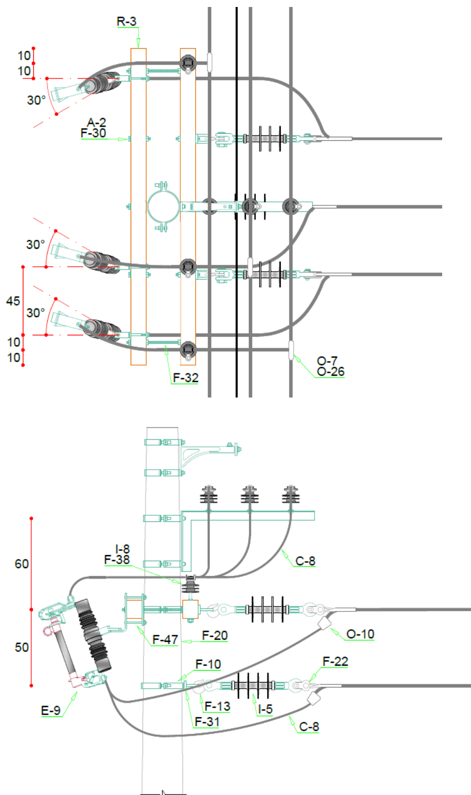
Figura 1 – Estrutura CE2H-CE3 CF Dimensões em cm
