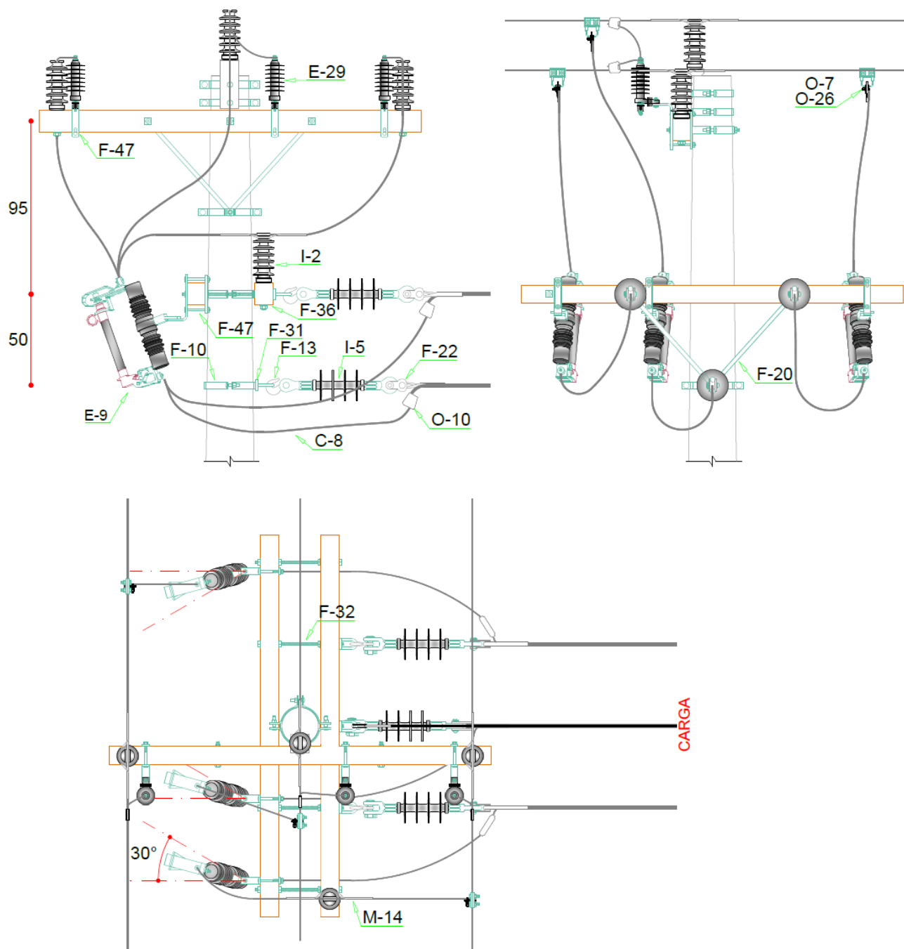
Figura 2 – Estrutura T1-CE3 CF Dimensões em cm
