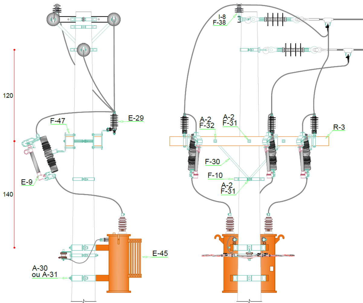
Figura 2 – Estrutura CE3U com transformador Dimensões em cm
