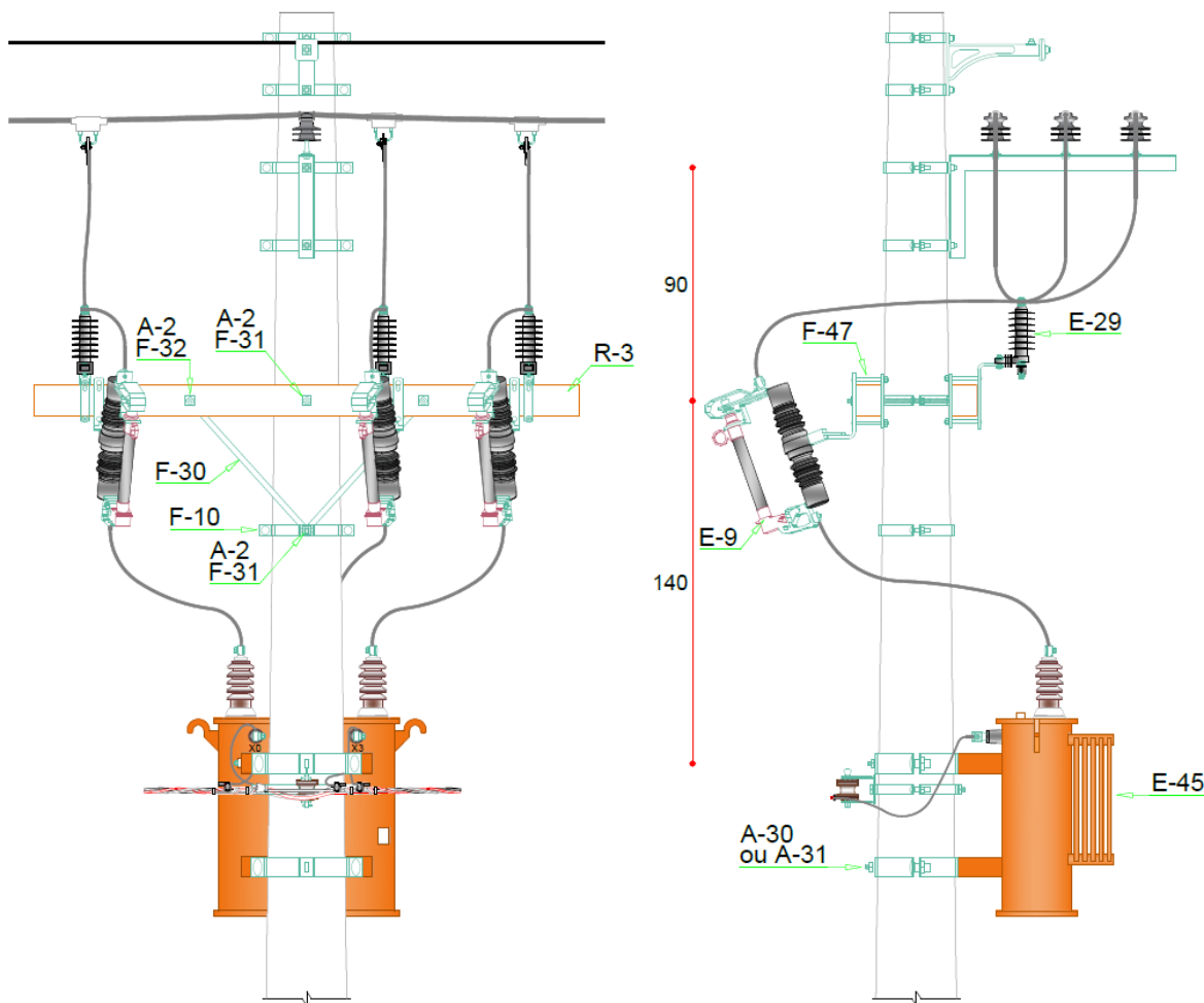
Figura 1 – Estrutura CE2H com transformador Dimensões em cm
