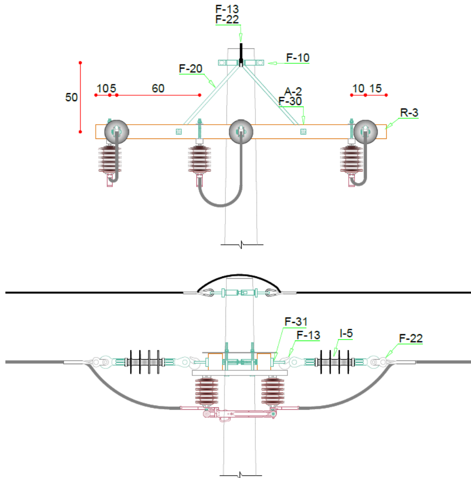
Figura 1 – Estrutura CE4 SU – 1º Nível Dimensões em cm
