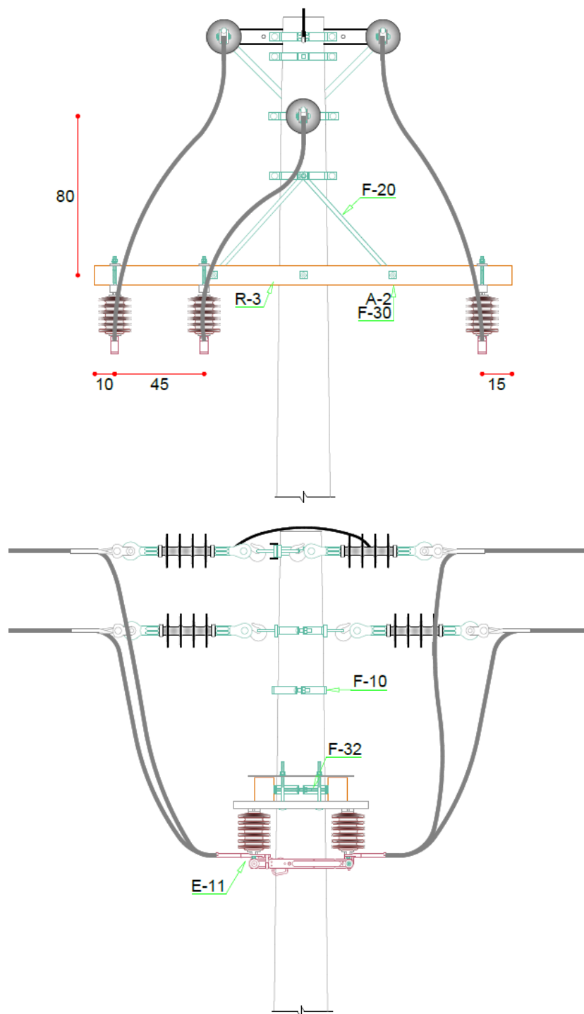
Figura 2 – Estrutura CE4U SU – 2º Nível Dimensões em cm
