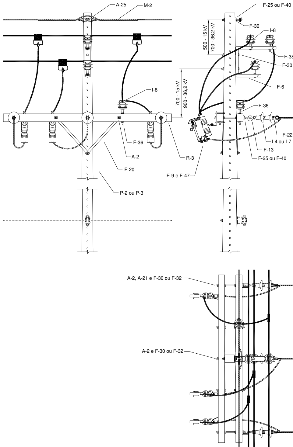
Figura 4 - Estrutura CE2-N3 CF – Poste de Concreto de Seção DT Dimensões em mm
